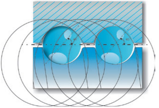
滚柱丝杠滚动体数目、曲率半径与滚珠丝杠滚动体接触面包络圆对比示意图
