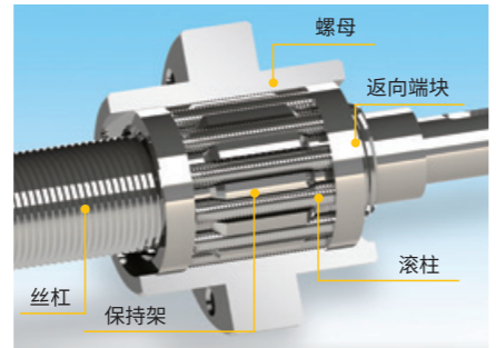
循环式行星滚柱丝杠副
