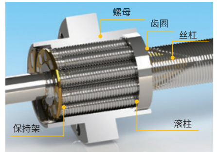
行星滚柱丝杠副
